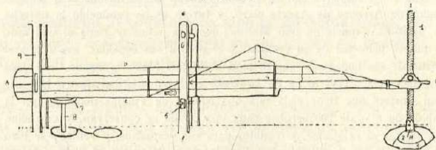
Fig. 17.—Viga de almazara: 1) husillo, 2) pesillo, 3) pesillo de abajo, 4) viga, 5) marrana, 6) guía, 7) plato, 8) telera, 9) bijerías, 10) reola. A-B = 14,30 m., B-C = 8,40 m., D-E = 1 m., F-G = 3,40 m., H-I = 4 m.
