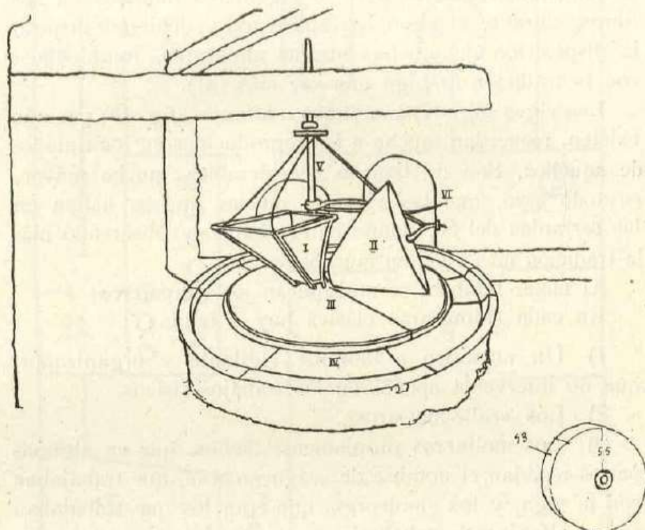
Fig. 18.—Muela de almazara: I) tolva, 1,25 m. de largo, 73 cms. de ancho hacia fuera, 63 hacia el eje; II) rulo, 1,3 m. de largo, 60 cms. de radio; III) solero (moledero y empiedro), 1,42 m. de radio, 60 cms. de altura; IV) alfanje (moledero y empiedro), 52 cm. de ancho, 60 cms. de altura; V) eje; VI) tiro.
