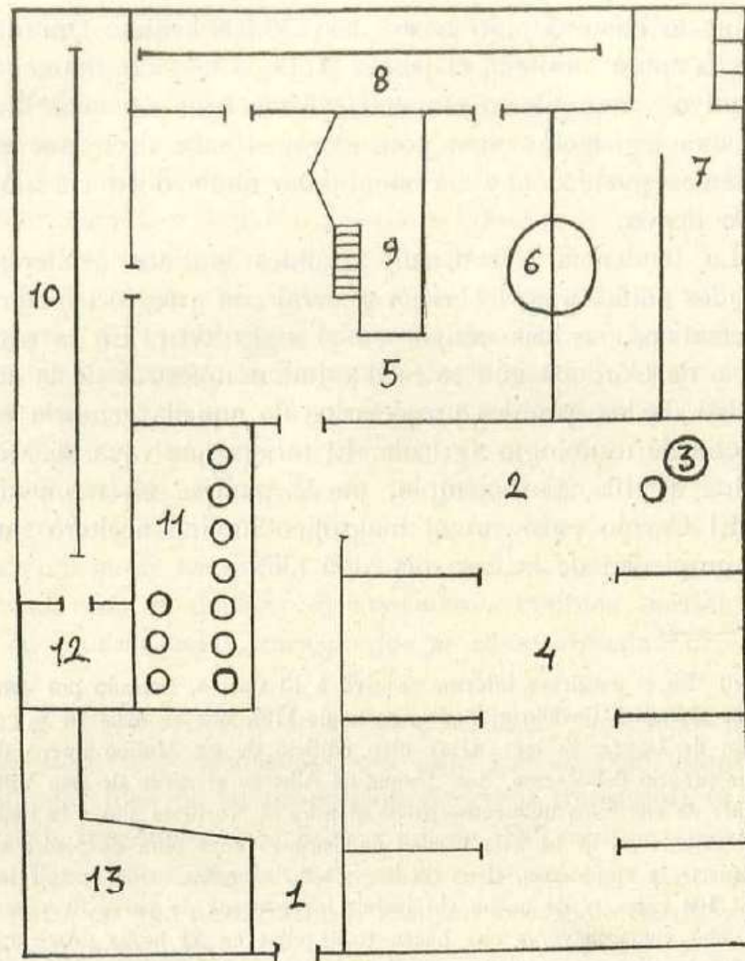
Fig. 16.—Plano de una almazara: 1) entrada, 2) patio (al aire libre), 3) pozos, 4) depósito de aceituna, 5) cuarto central, 6) tolva, 7) cuadra, 8) viga primera, 9) cocina, 10) viga segunda, 11) tinajas, 12) depósito, 13) casilla.
